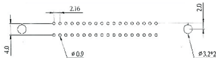
P.C.BOARD LAYOUT
